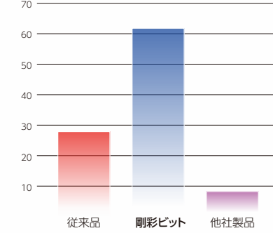
打ち込み試験 木材への打ち込み N=5 (本)
