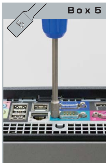
M2.5 ネジのナットに使える 対辺 5mm のソケット差替軸。
