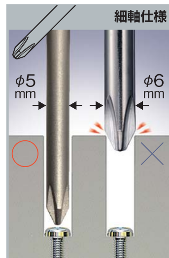
軸径 5mm の細軸仕様で電気製品などの 分解に便利。
