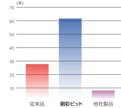
打ち込み試験 木材への打ち込み N=5
